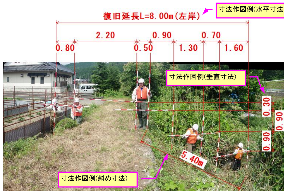
寸法作図例
